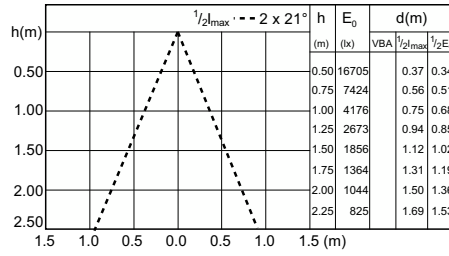
Beam diagram - CDM-Rm Elite Mini 35W/930 GX10 MR16 40D
