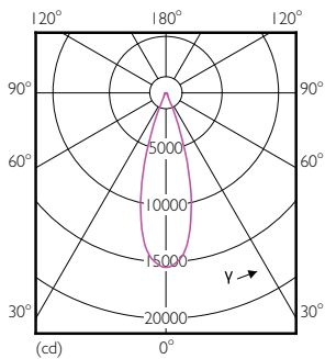
LEDspot E27 PAR30L 40W 6000K
